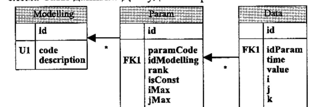
Рис. 1. Обобщенная схема базы данных для хранения численных результатов вычислительных экспериментов
