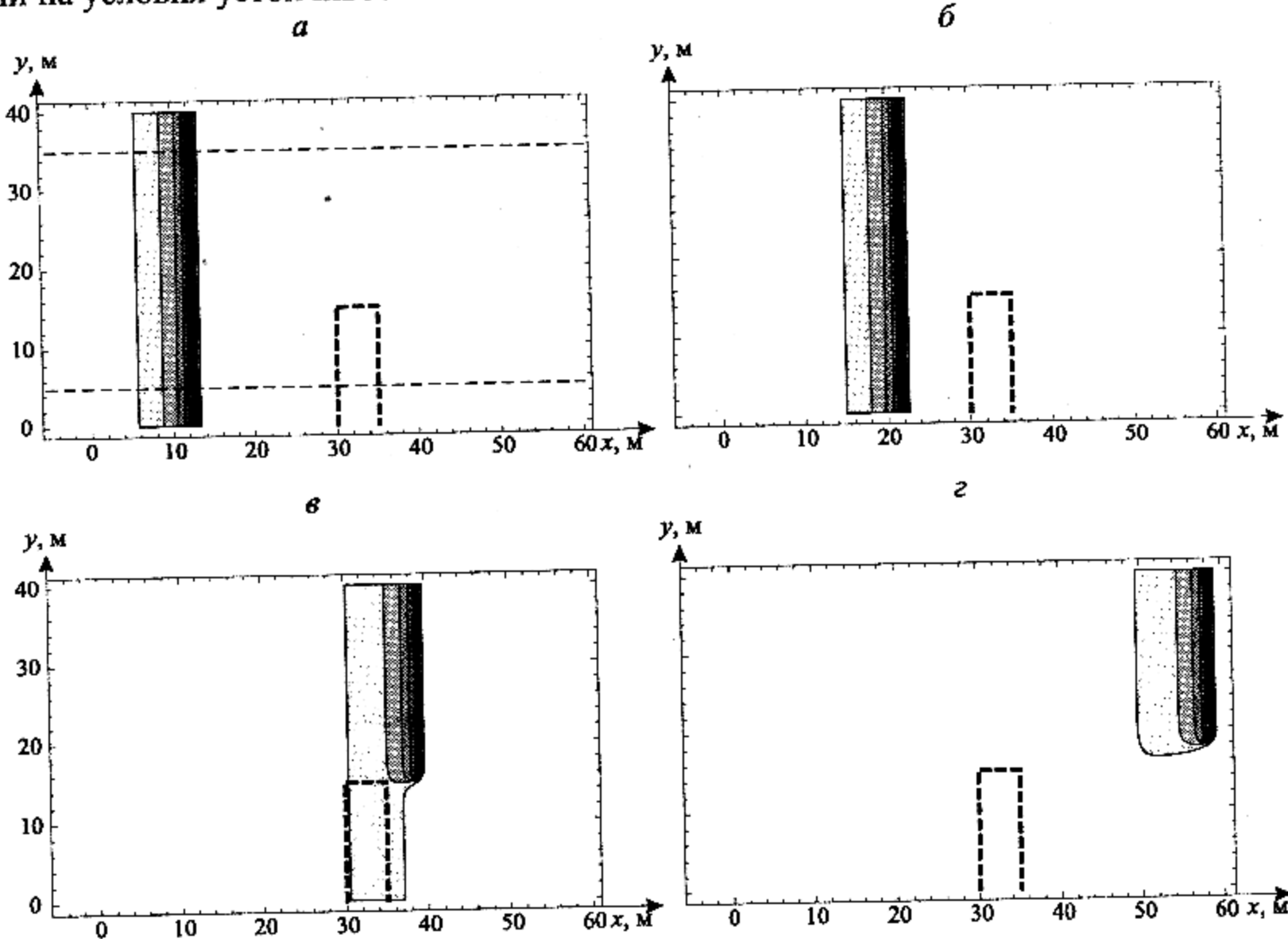
Рис. 2. Карты изолиний температуры во фронте верхового пожара (вид сверху) в случае неоднородного распределения лесных горючих материалов в моменты времени: а - 1,5, б - 3, в - 6, г - 9 с
